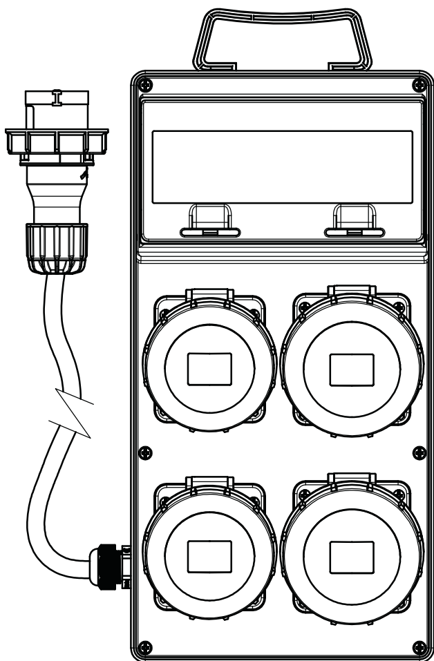
Figura 1 costruzione e figura del quadro di distribuzione tipo 94677
