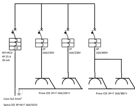
Figura 2 ----- configurazione dello schema elettrico
